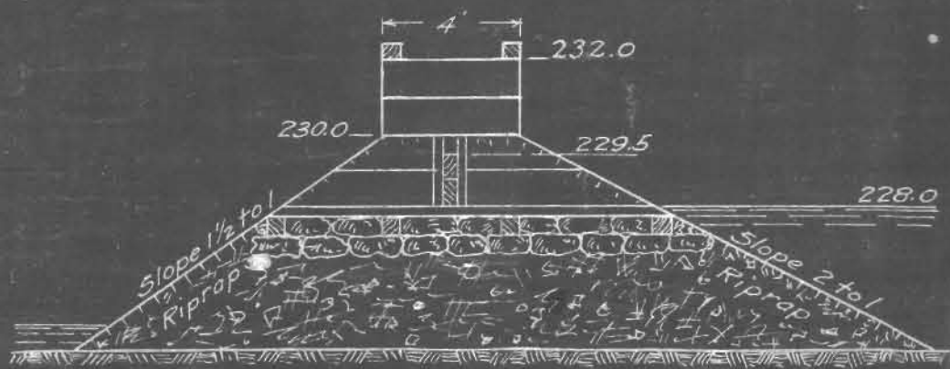
SECTION A-B
