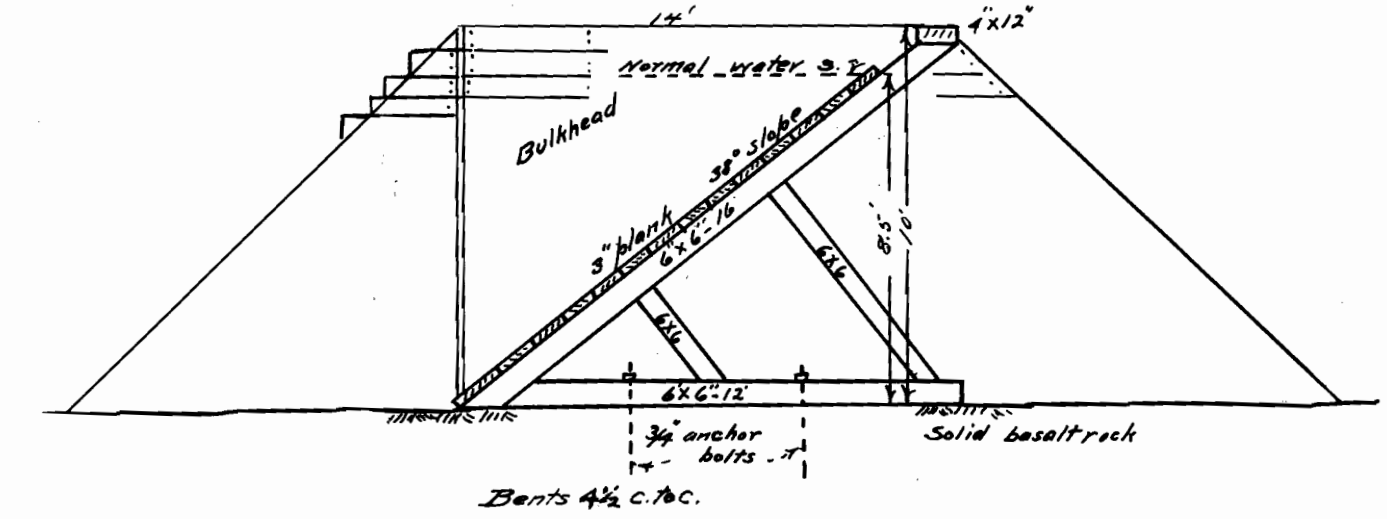
DIVERSION DAM.
