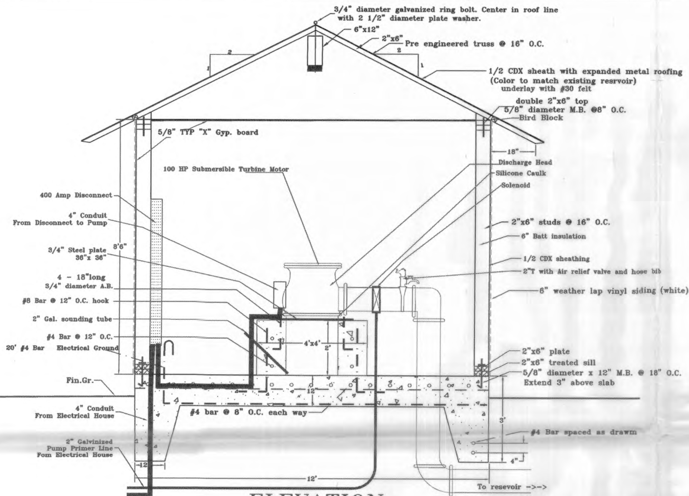
ELEVATION
